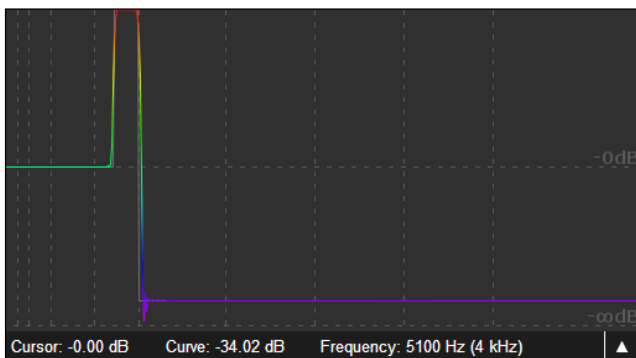
Figura 4. Ondulação da resposta em frequência devido à alterações bruscas de ganho.
